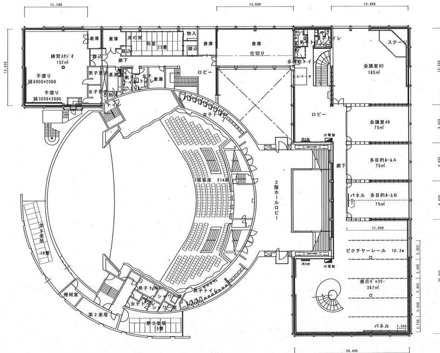
2階 平面図
