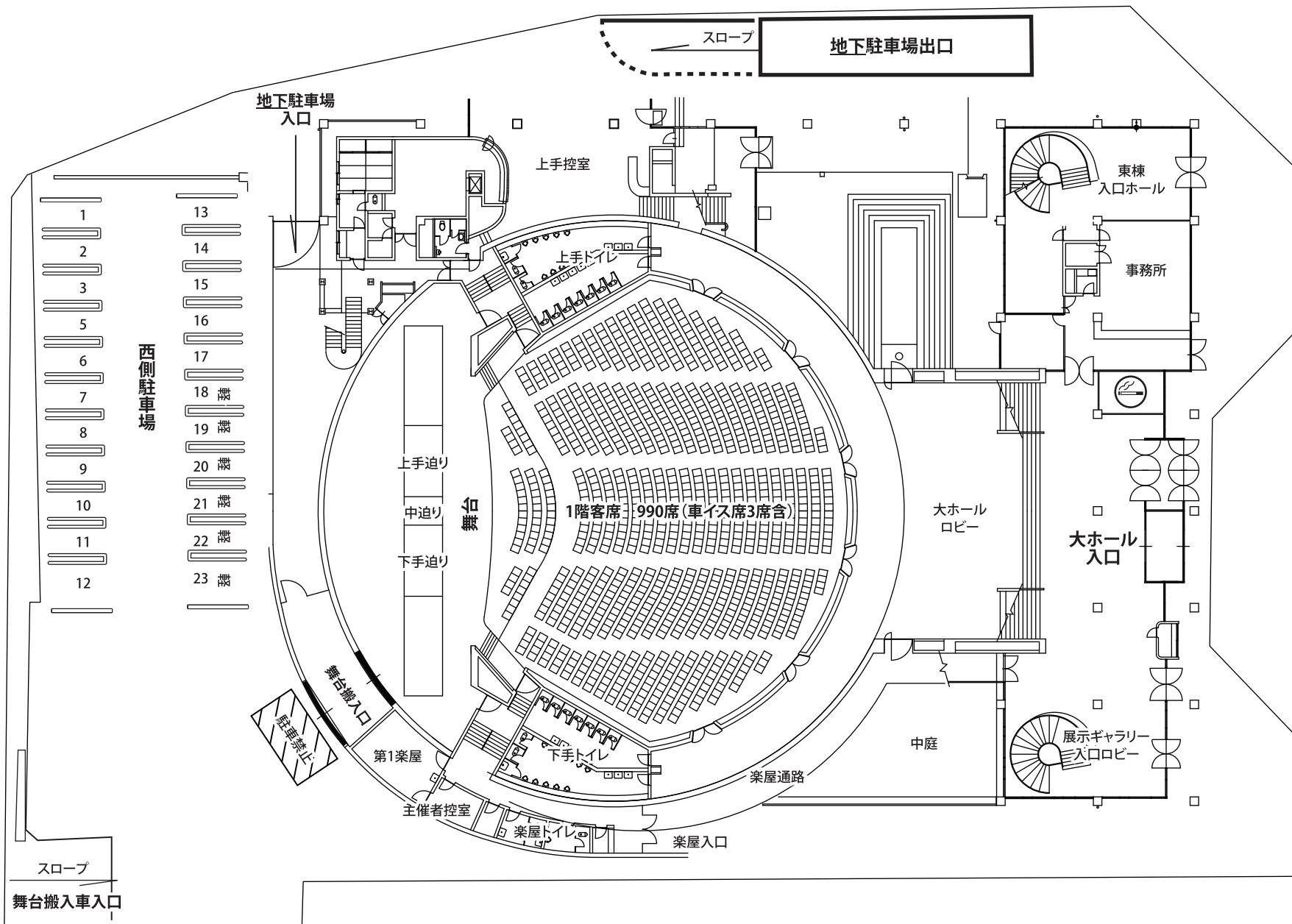
1階平面図
