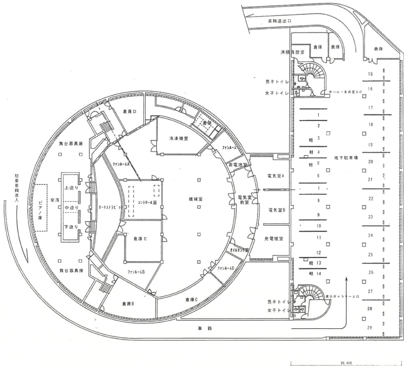
B1階 平面図
